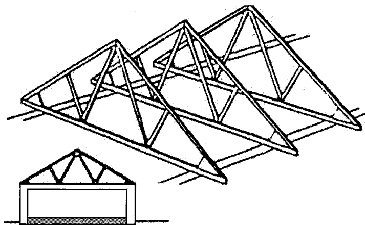
Croquis 16
