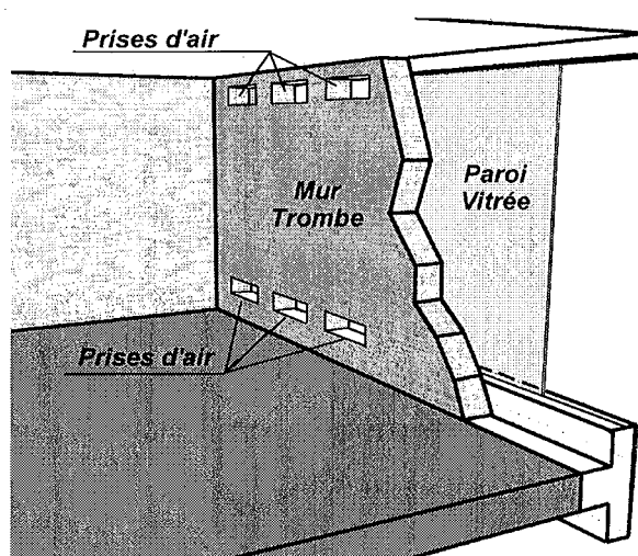
Croquis 7
