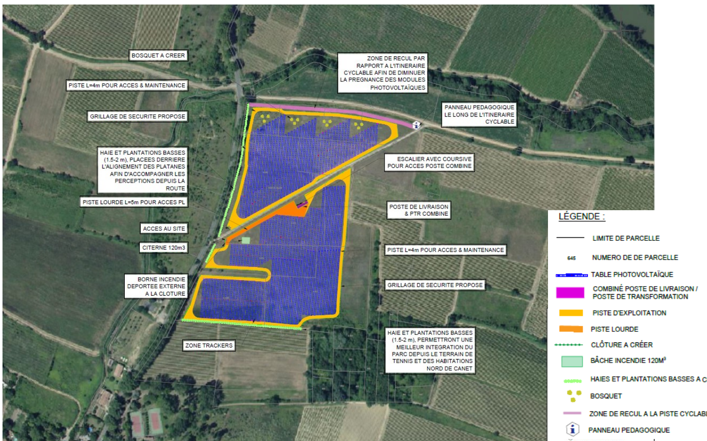
Figure 2 : plan des principaux équipements du projet – source BD ortho IGN 1/2500 réalisation TotalEnergies
