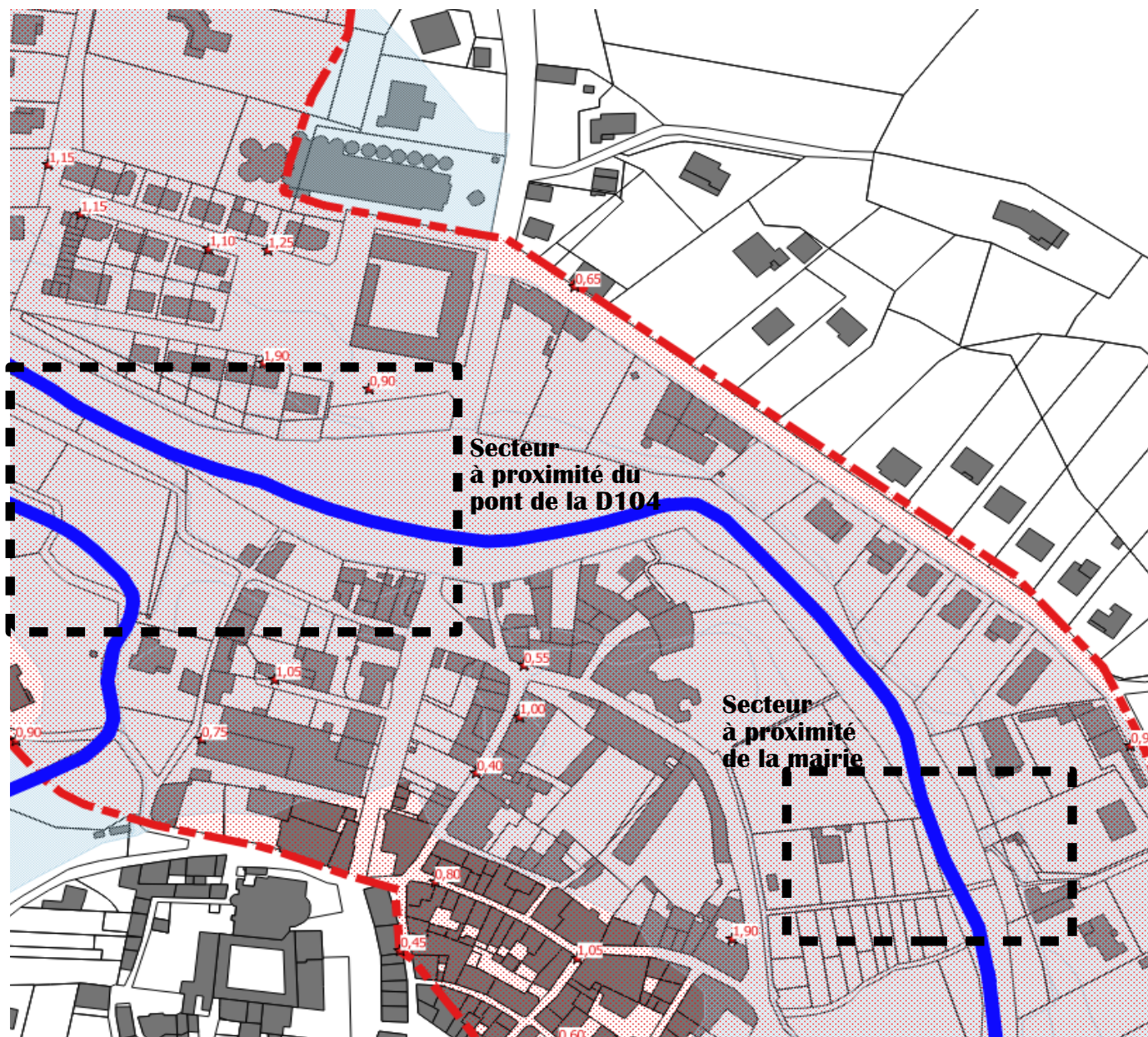
Carte de l'emprise inondée le 15 octobre 2018 à Saint-Hilaire, ainsi que les hauteurs d'eau relevées- Extrait.
