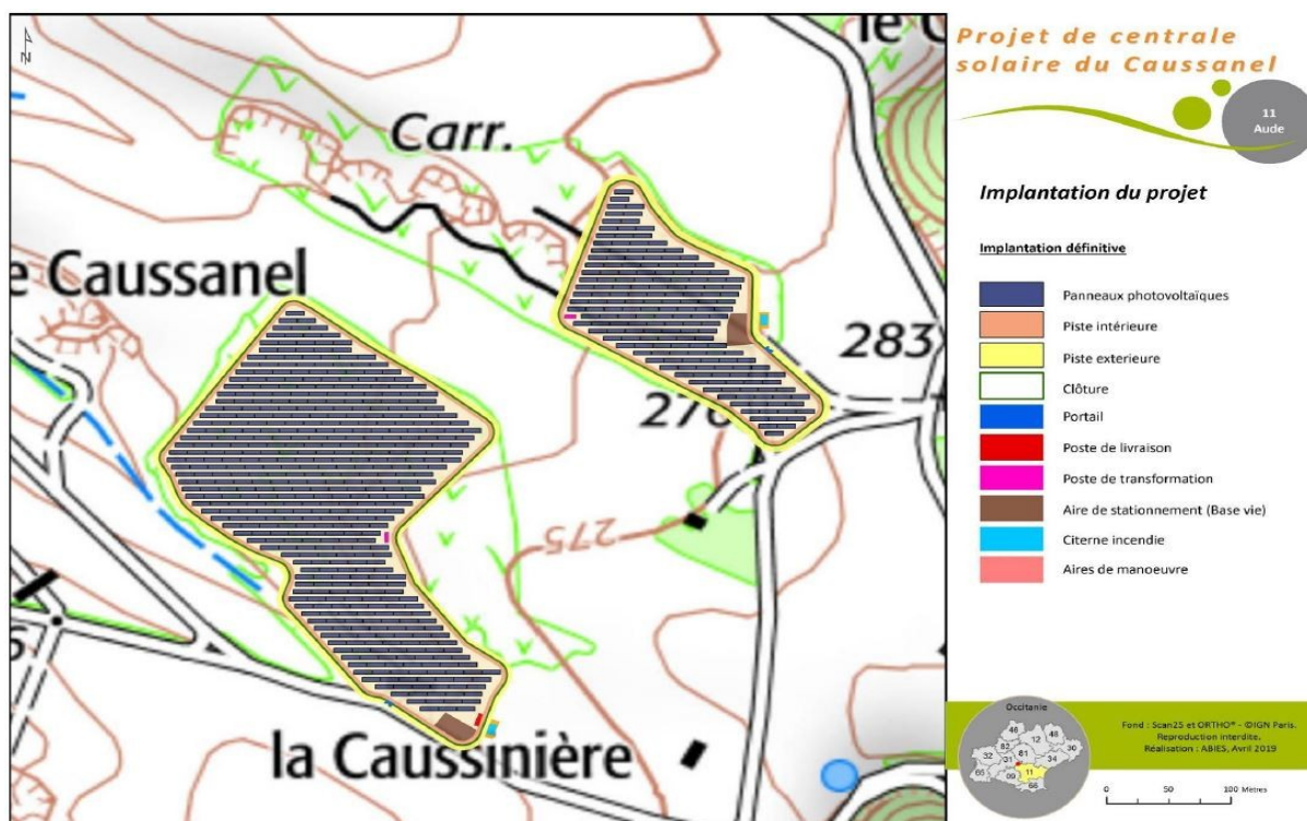
Figure 2: Plan de masse
