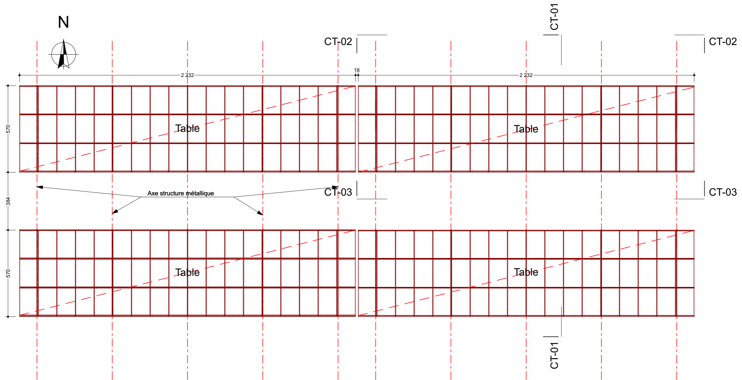
0. Plan Table photovoltaïque 1:150
