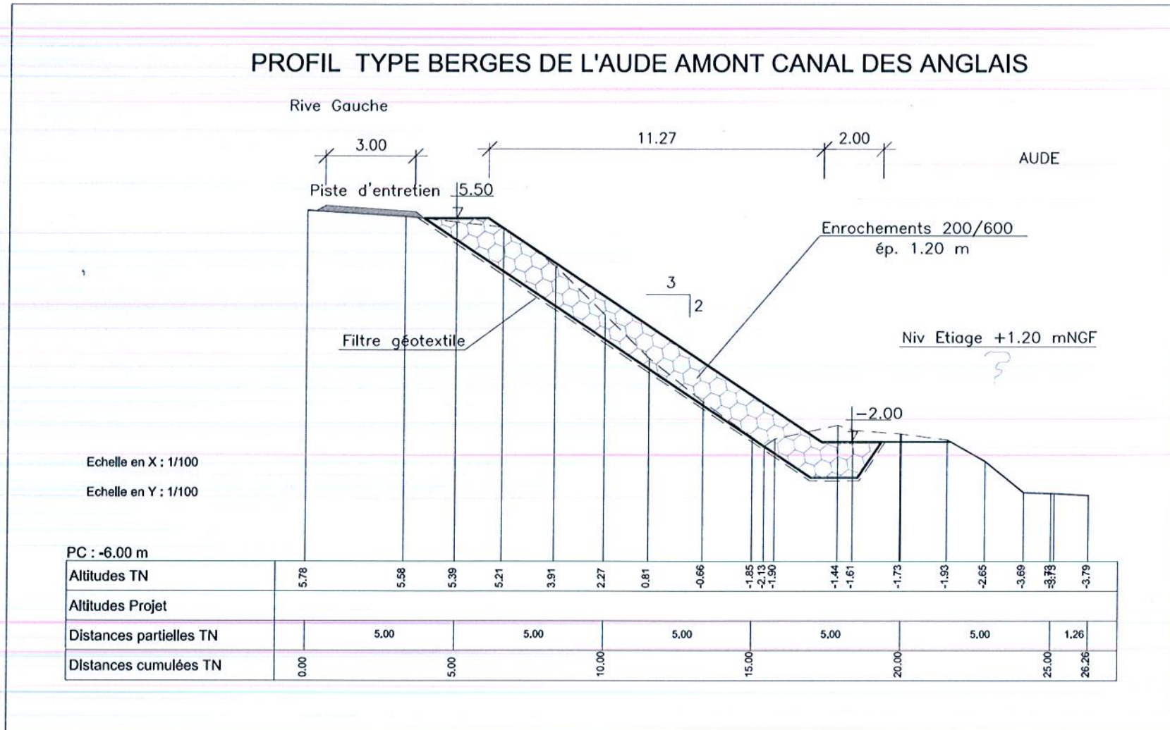
Figure 8 : Profil type aménagement des berges de l'Aude en amont du canal des Anglais
