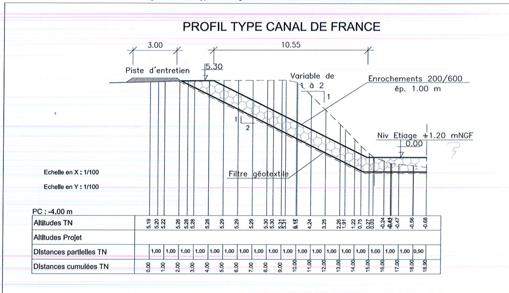
Figure 7 : Profil type aménagement de l'exutoire du canal de France
