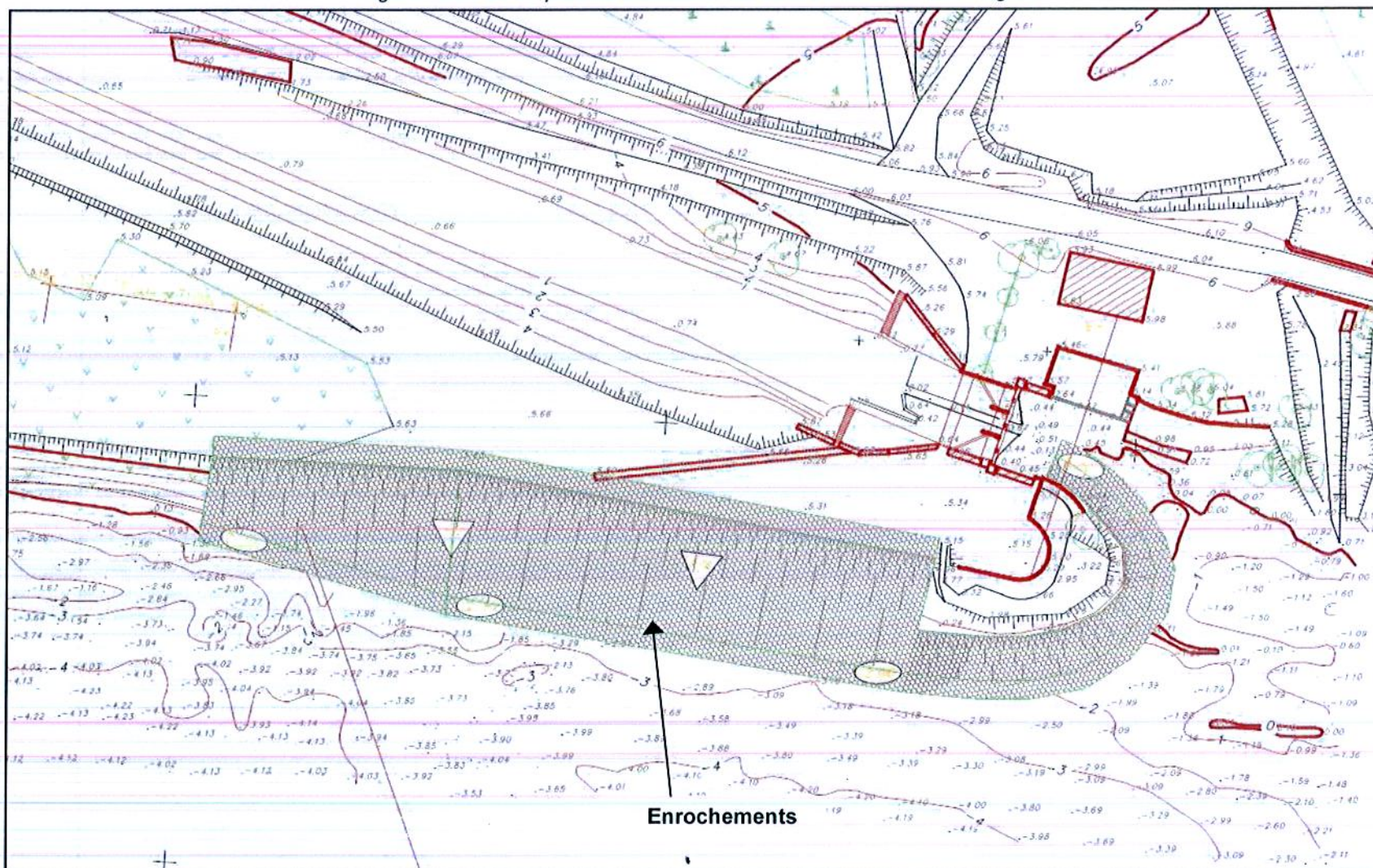
Figure 10 : Vue en plan du confortement au droit du canal des Anglais
